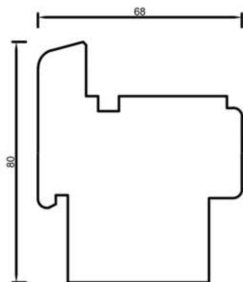
68154 Rama 80 mm
