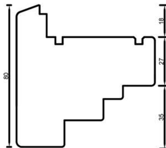
78306 Poprzeczka 80 mm
