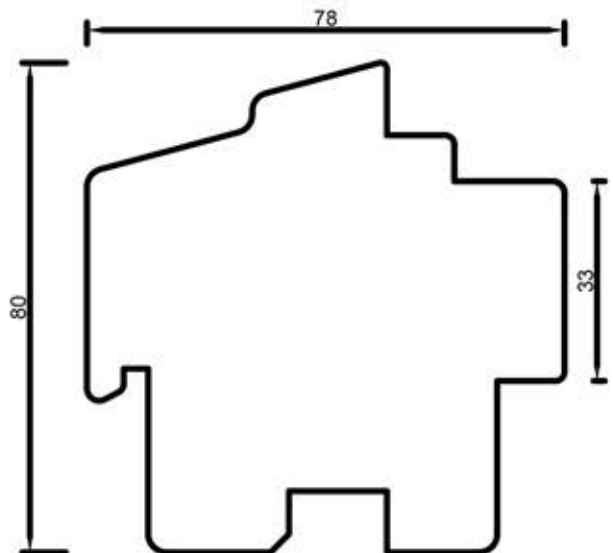
78112 Rama 80 mm
