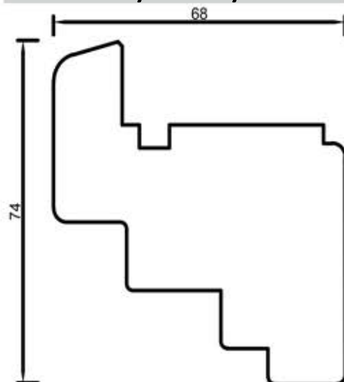
68258 Fałszywe skrzydło 74 mm
