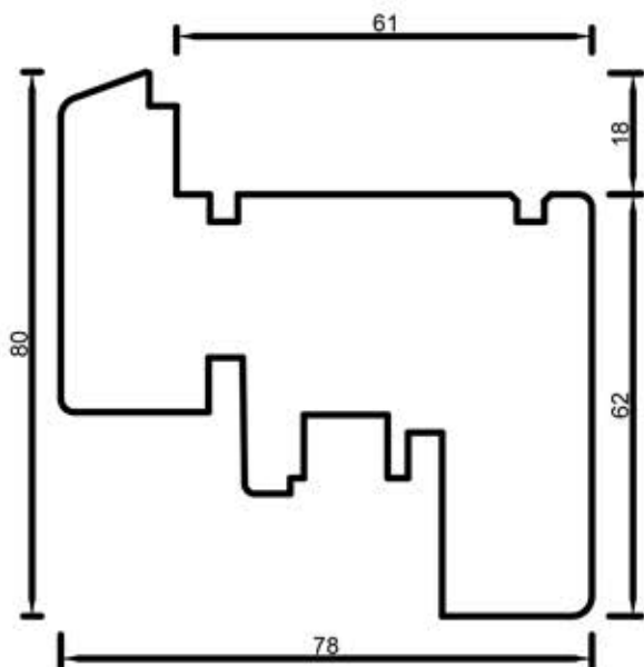
78201 Skrzydło 80 mm
