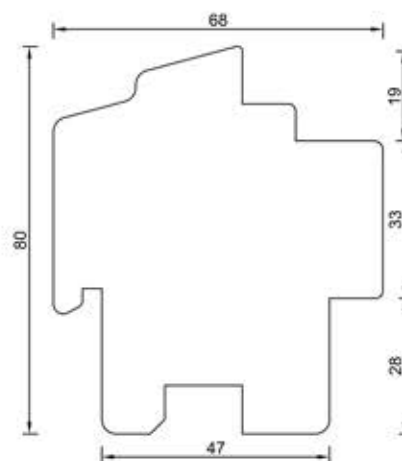
68122 Rama 80 mm
