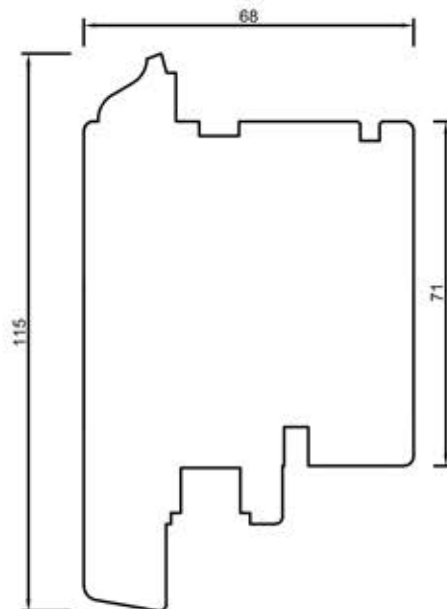
68212 Skrzydło T 115 mm
