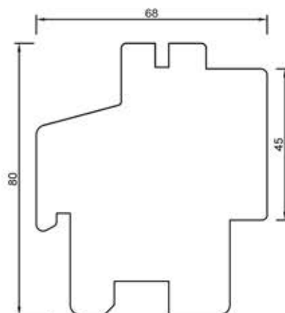
68102 Rama 80 mm
