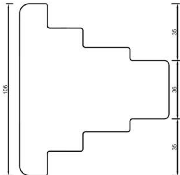
92301 Słupek stały 106 mm
