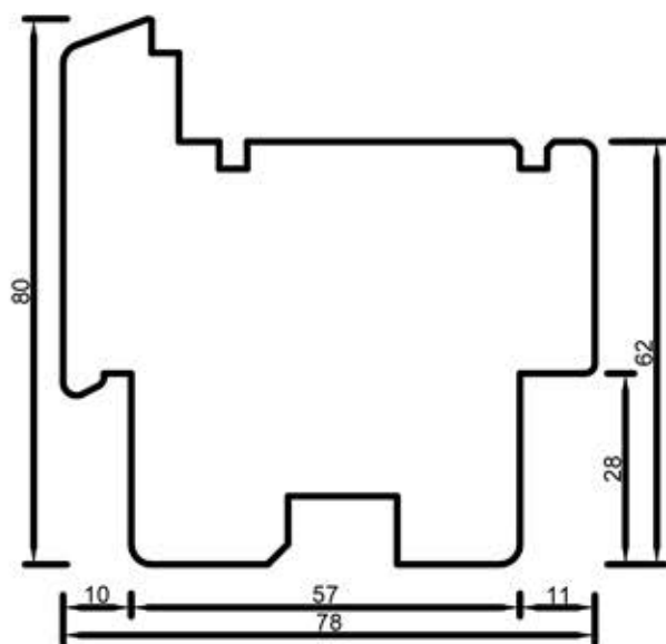
78104 Rama 80 mm
