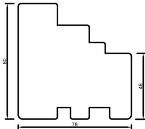
78101 Rama 80 mm
