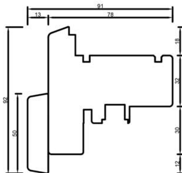
78401 Stulp 50 mm
