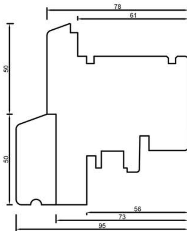
78208 Skrzydło 100 mm
