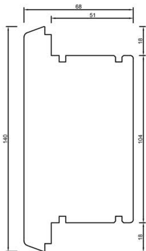
68303 Słupek stały 140 mm
