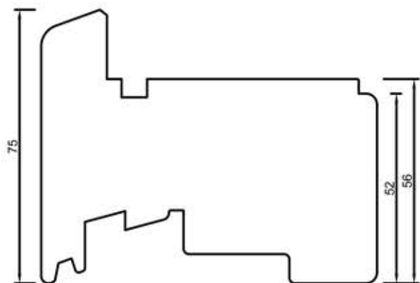
92209 Fałszywe skrzydło 75 mm
