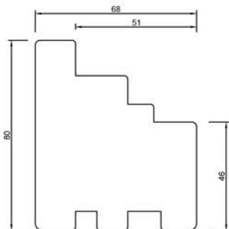
68101 Rama 80 mm
