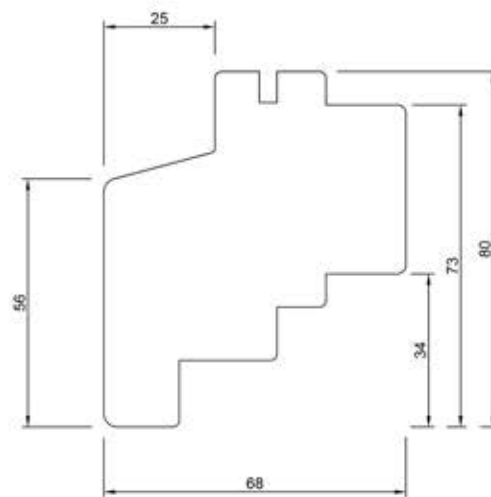
68302 Poprzeczka 80 mm
