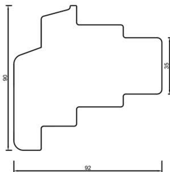
92302 Poprzeczka 90 mm
