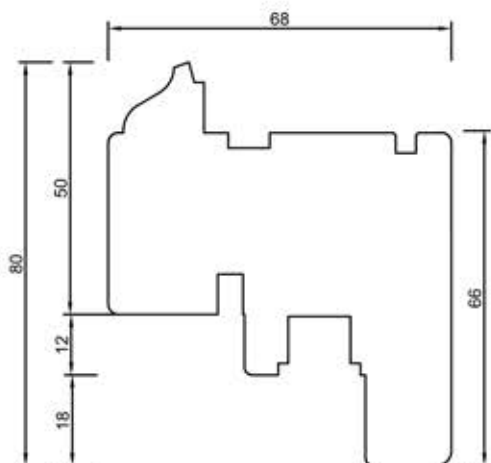
68211 Skrzydło 80 mm
