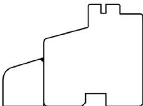
68143 Rama 80 mm
