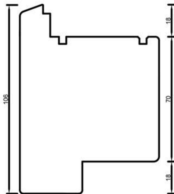
78307 Poprzeczka 106 mm
