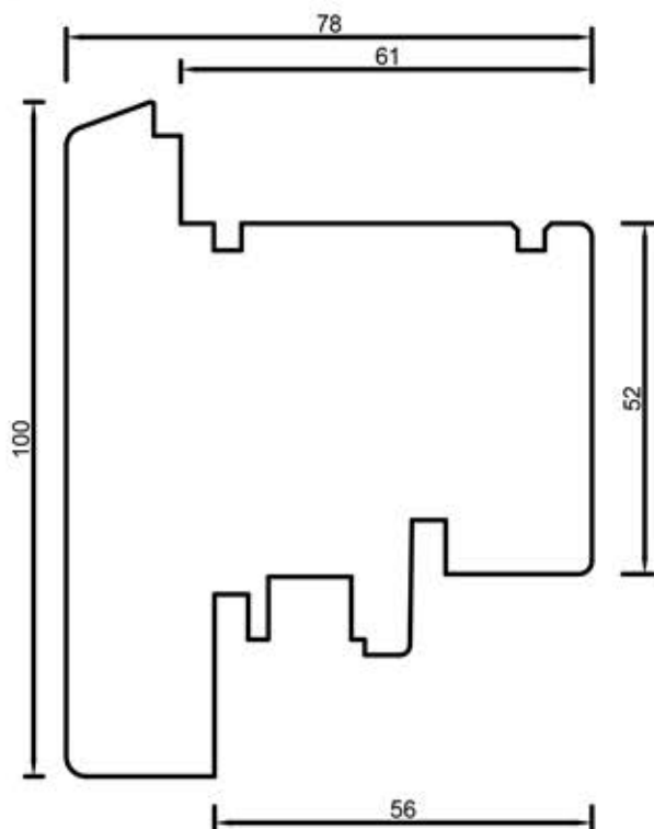
78207 Skrzydło 100 mm
