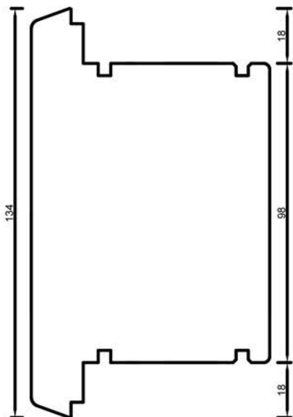
78303 Słupek stały 134 mm
