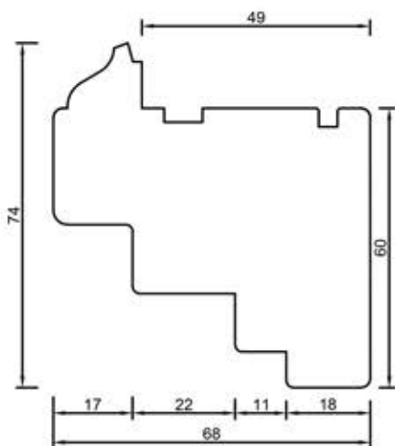
68219 Fałszywe skrzydło 80 mm
