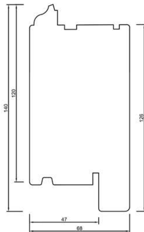
68213 Skrzydło 140 mm
