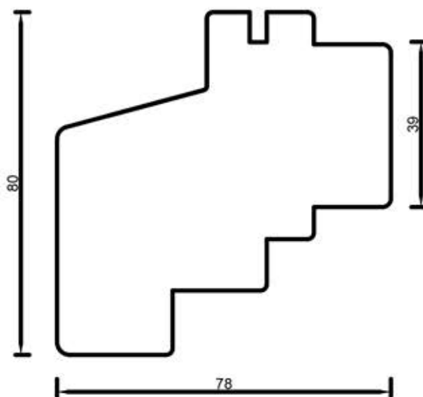
78302 Poprzeczka 80 mm
