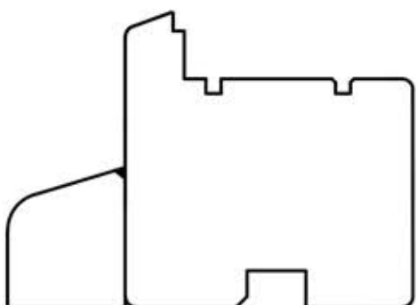
68145 Rama 80 mm
