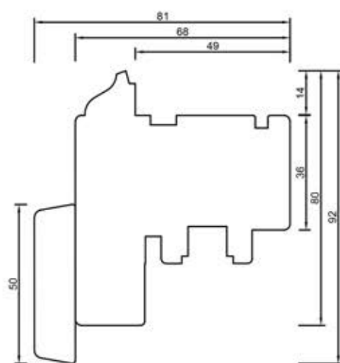
68411 Stulp 50 mm
