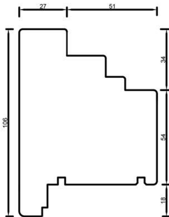
78305 Poprzeczka 106 mm
