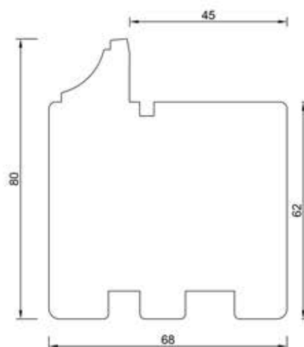
68123 Rama 80 mm
