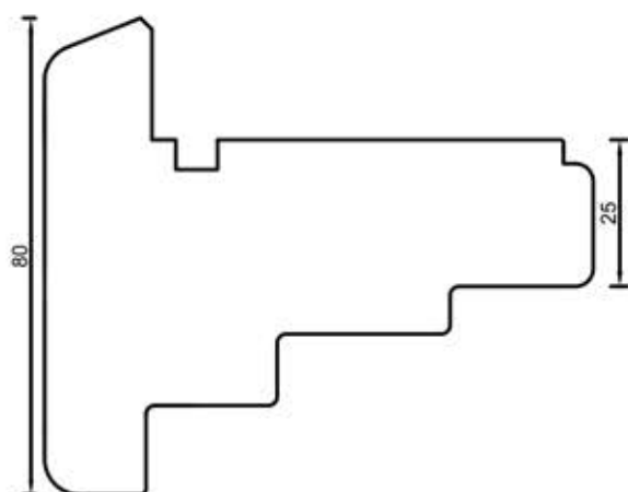
92303 Poprzeczka 80 mm
