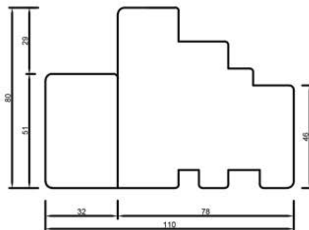
68144 Rama 80 mm
