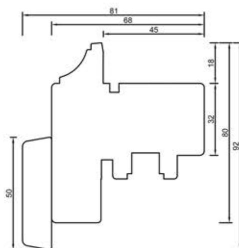
68421 Stulp 50 mm
