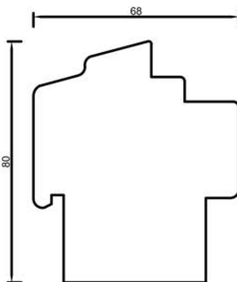
68155 Rama 80 mm
