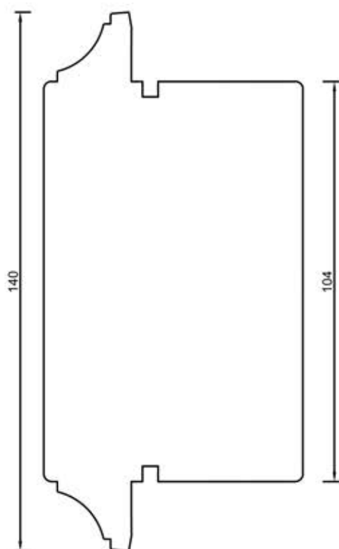
68323 Słupek stały 140 mm
