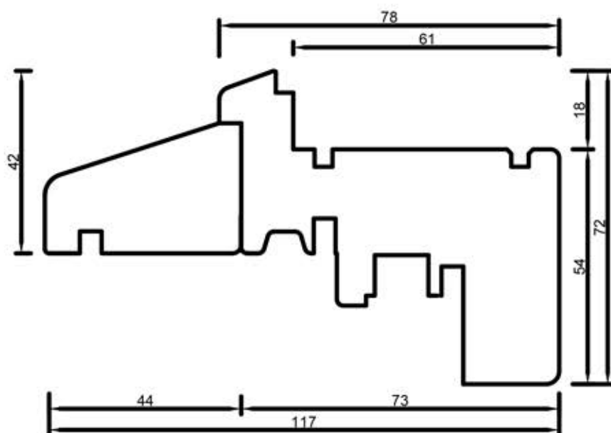
78212 Skrzydło 72 mm
