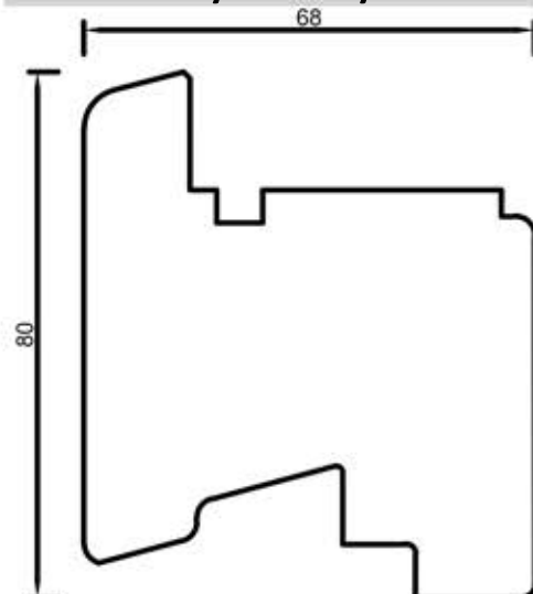
68259 Fałszywe skrzydło 80 mm
