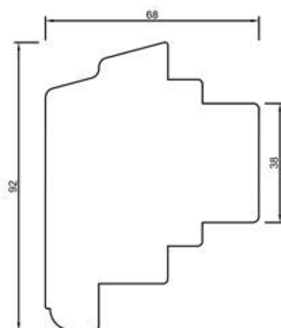
68324 Poprzeczka 80 mm
