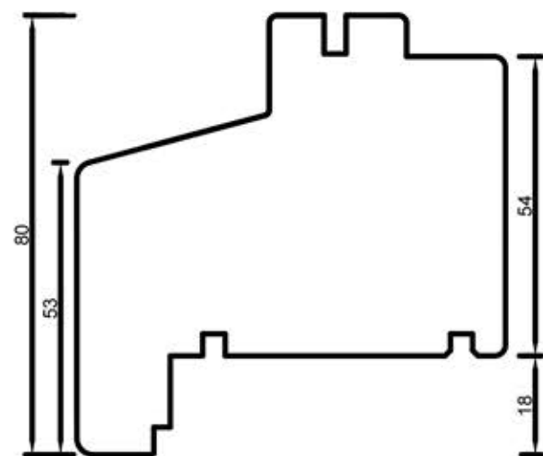
78304 Poprzeczka 80 mm
