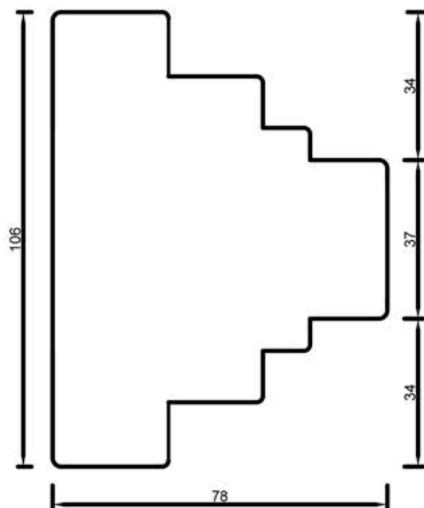
78301 Słupek stały 106 mm
