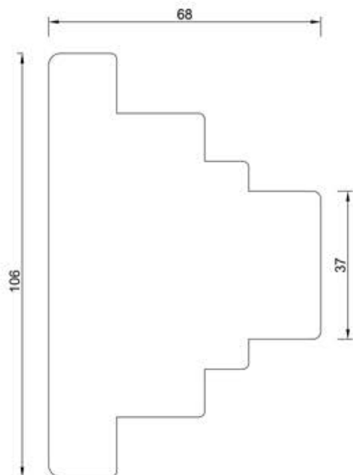
68301 Słupek stały 106 mm
