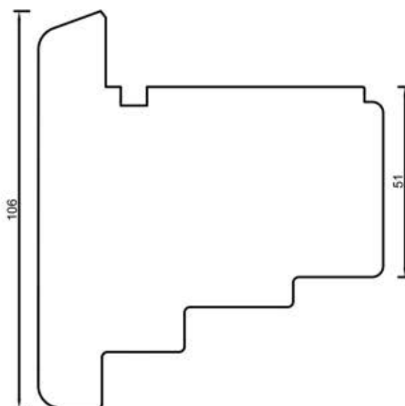
92304 Poprzeczka 106 mm
