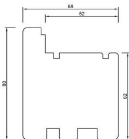
68103 Rama 80 mm
