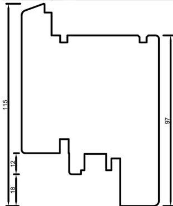
78205 Skrzydło tarasowe 115 mm
