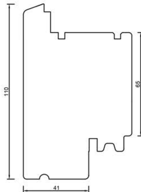
68206 - Dolny profil skrzydła 68205
