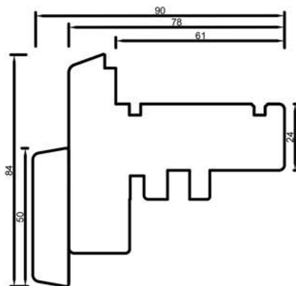
78411 Stulp 50 mm
