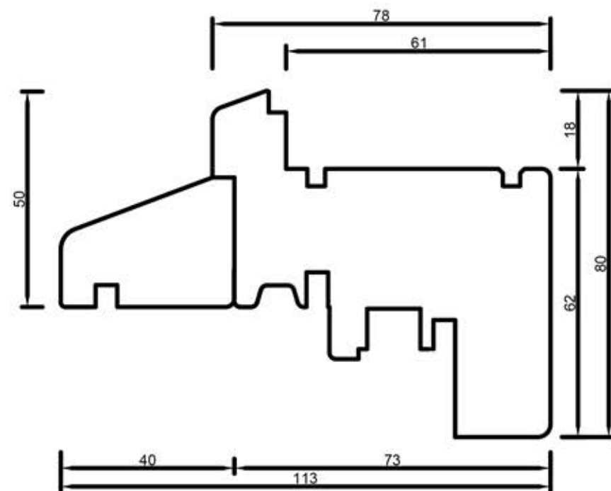
78211 Skrzydło 80 mm
