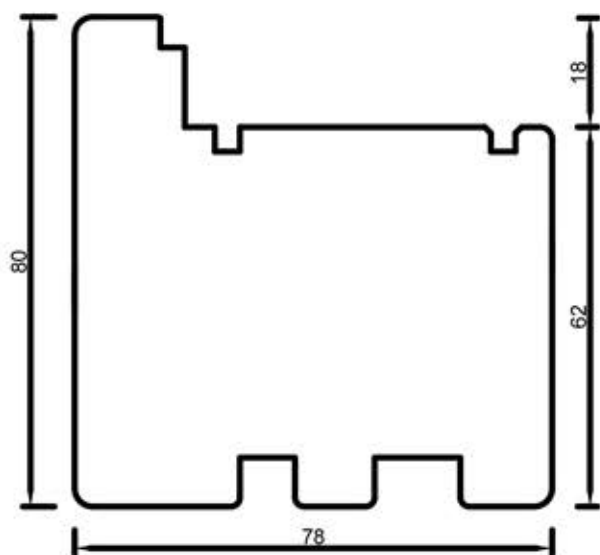
78103 Rama 80 mm
