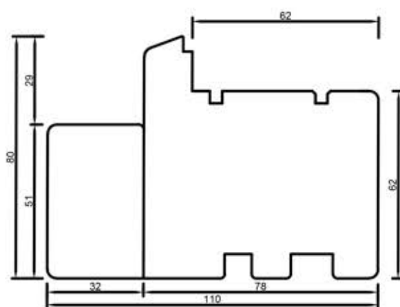
68144 Rama 80 mm
