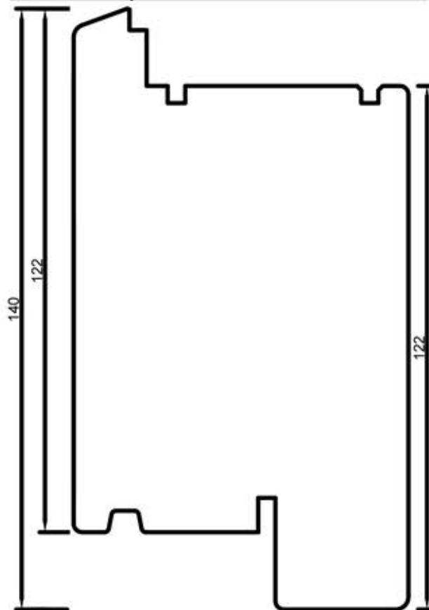
78206 Skrzydło drzwiowe 140 mm
