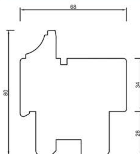
68124 Rama 80 mm
