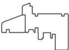
78211 Skrzydło 80 mm Strona 42
