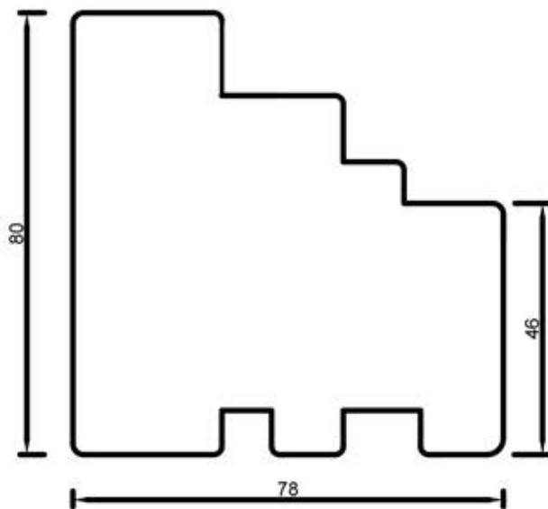
78111 Rama 80 mm
