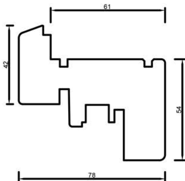
78213 Skrzydło 72 mm
