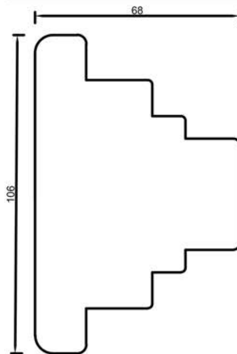
68351 Słupek stały 106 mm
