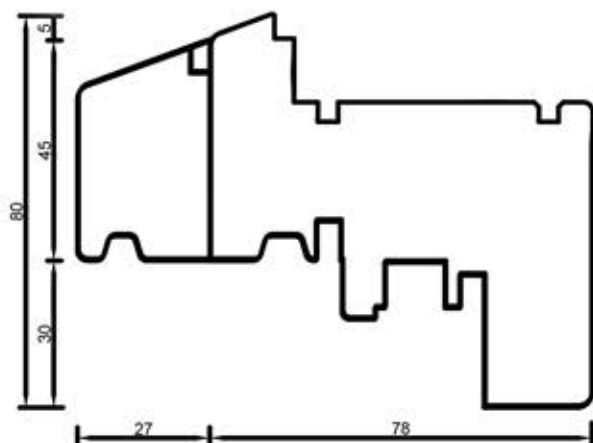
78203 Skrzydło balkonowe 80 mm
