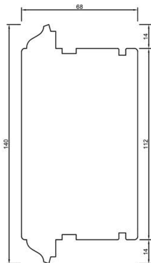
68313 Słupek stały 140 mm
