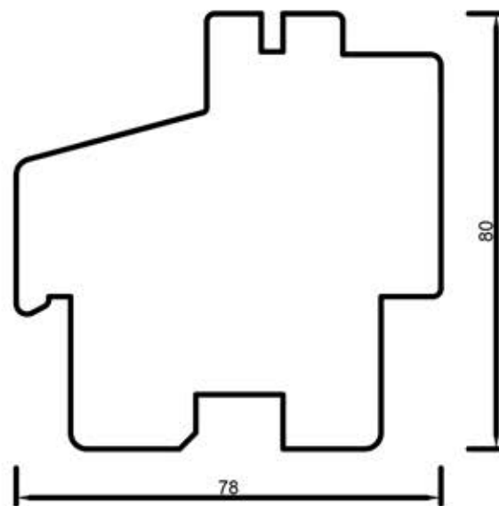
78102 Rama 80 mm
