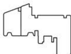
78203 Skrzydło 80 mm Strona 35
