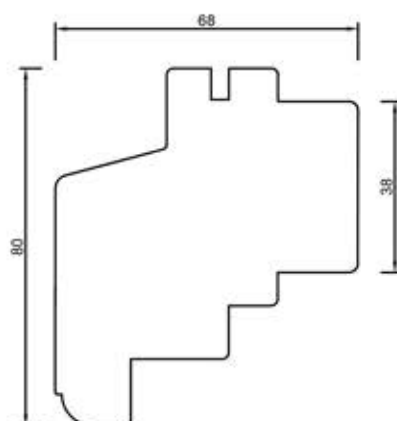
68322 Poprzeczka 80 mm
