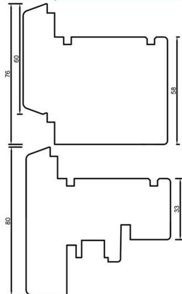
78209 Skrzydło 80 mm, 78809
