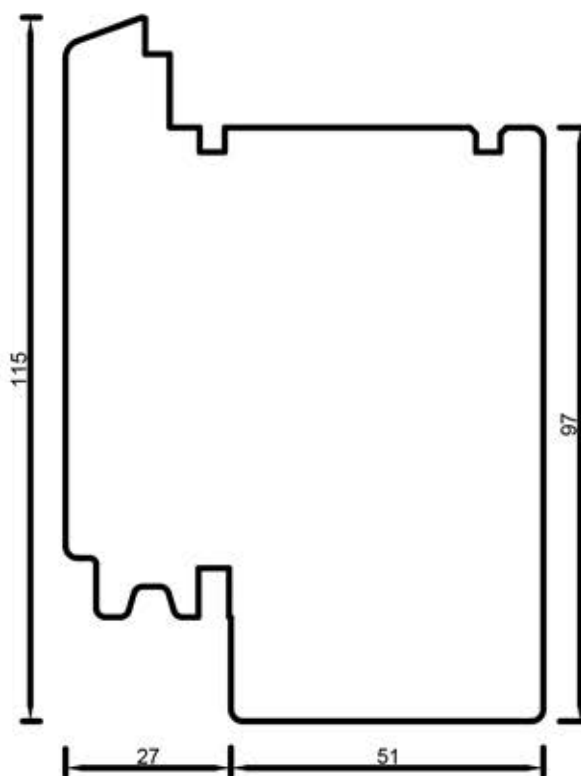
78204 Skrzydło tarasowe 115 mm
