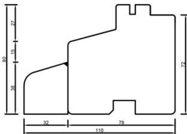
68141 Rama 68 mm
