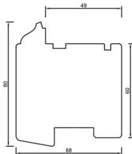
68219 Fałszywe skrzydło 80 mm
