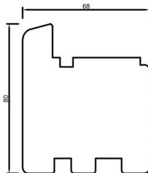
68153 Rama 80 mm
