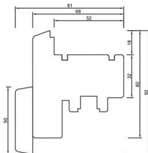
68401 Stulp 50 mm
