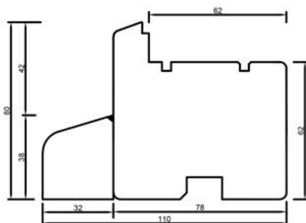
68141 Rama 68 mm
