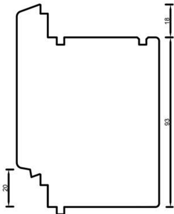
78802 111 mm
