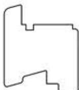
68259 Fałszywe skrzydło 80 mm Strona 27
