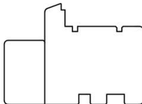
68144 Rama 80 mm
