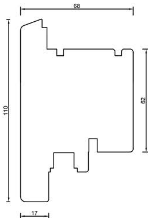
68205 Skrzydło T 110 mm
