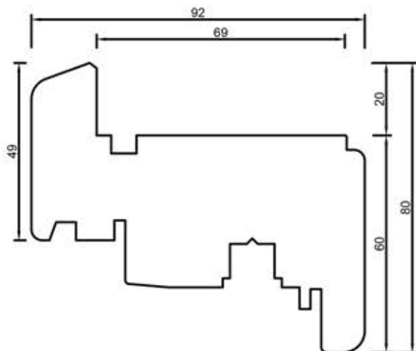
92201 Skrzydło 80 mm
