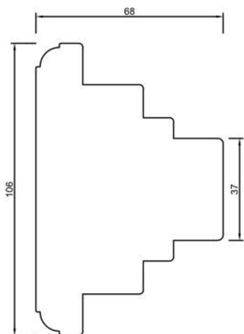
68321 Słupek stały 106 mm
