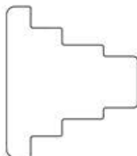
92301 Słupek 106 mm Strona 58
