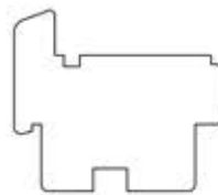
92104 Rama 80 mm Strona 55
