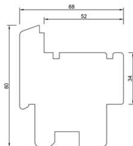
68104 Rama 80 mm
