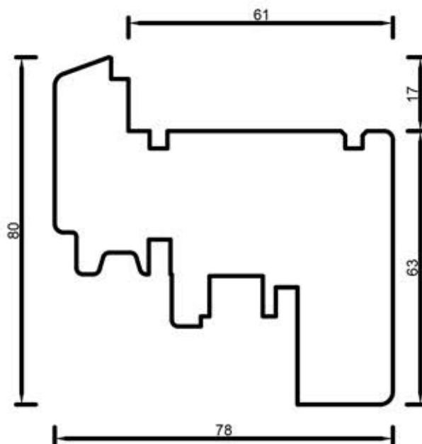
78202 Skrzydło 80 mm
