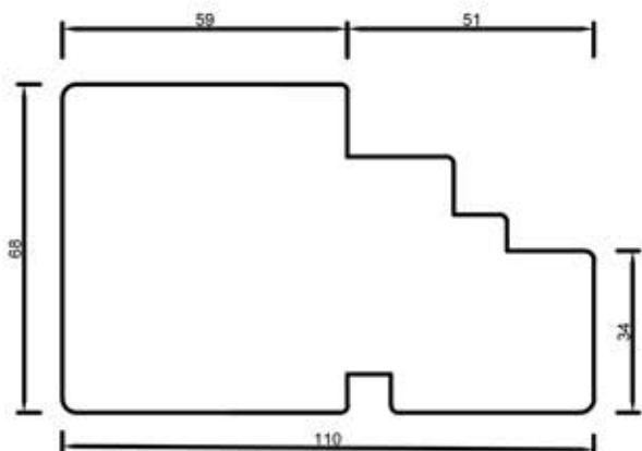
68141 Rama 68 mm
